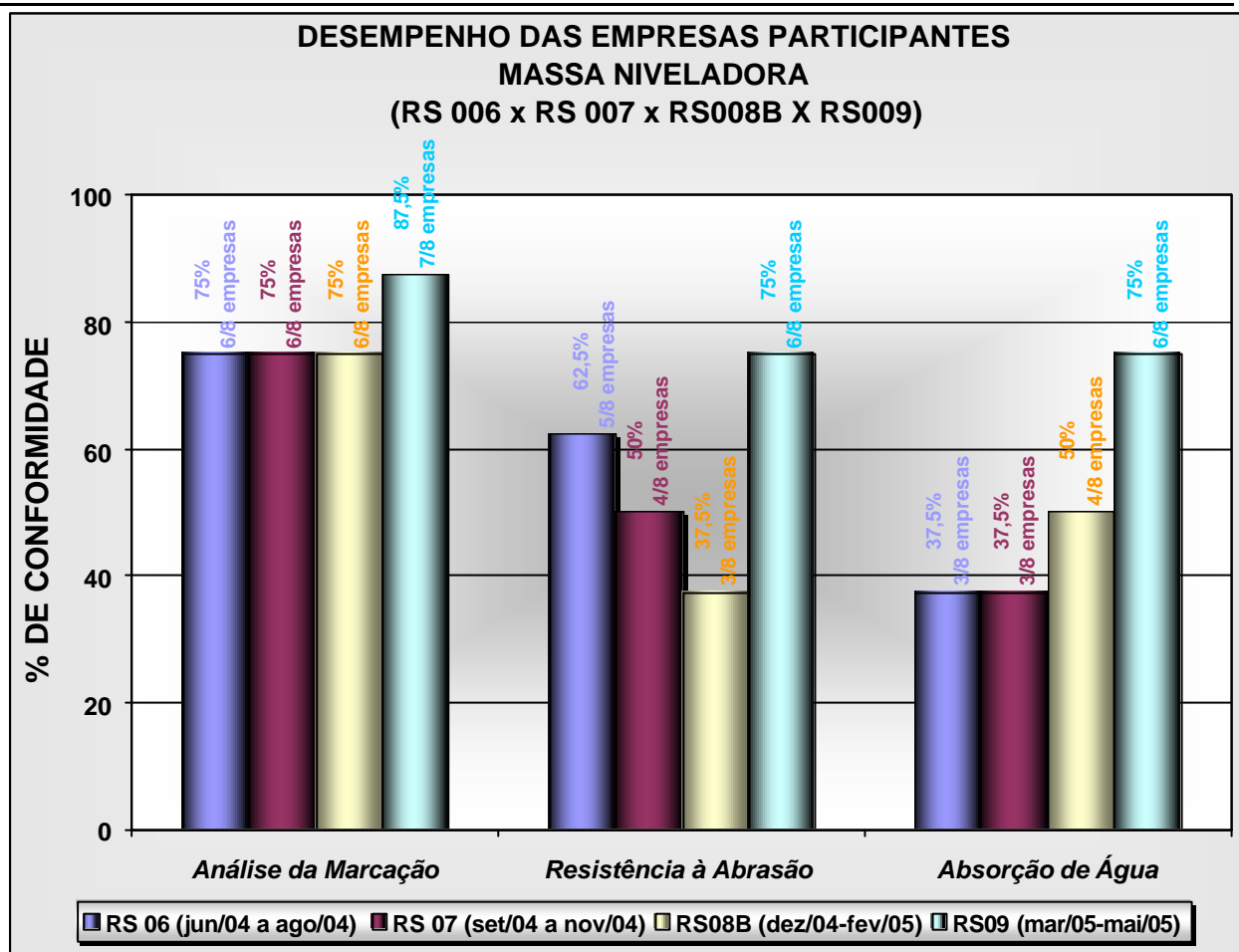
Figura 3 - Evolução das empresas PARTICIPANTES para cada análise realizada nas massas niveladoras no âmbito do Programa de Qualidade
