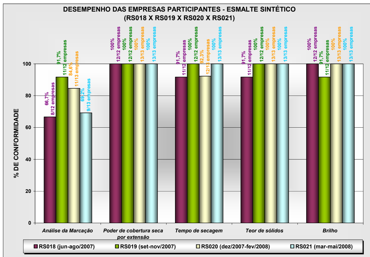
Figura 7 - Evolução das empresas PARTICIPANTES para cada análise realizada nos esmaltes sintéticos no âmbito do Programa de Qualidade
